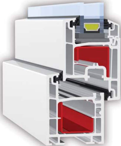
3-Kammer-Anschlagdichtungssystem mit 58mm Bautiefe
